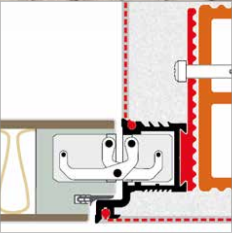
SEZIONE TELAIO DI SERIE
